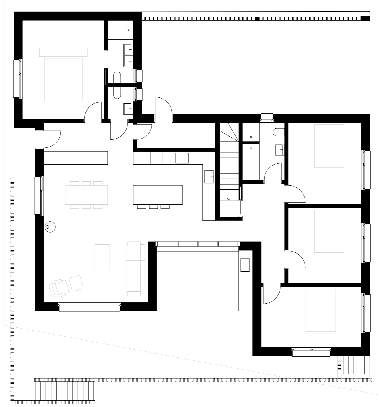
rez-de-chaussée
